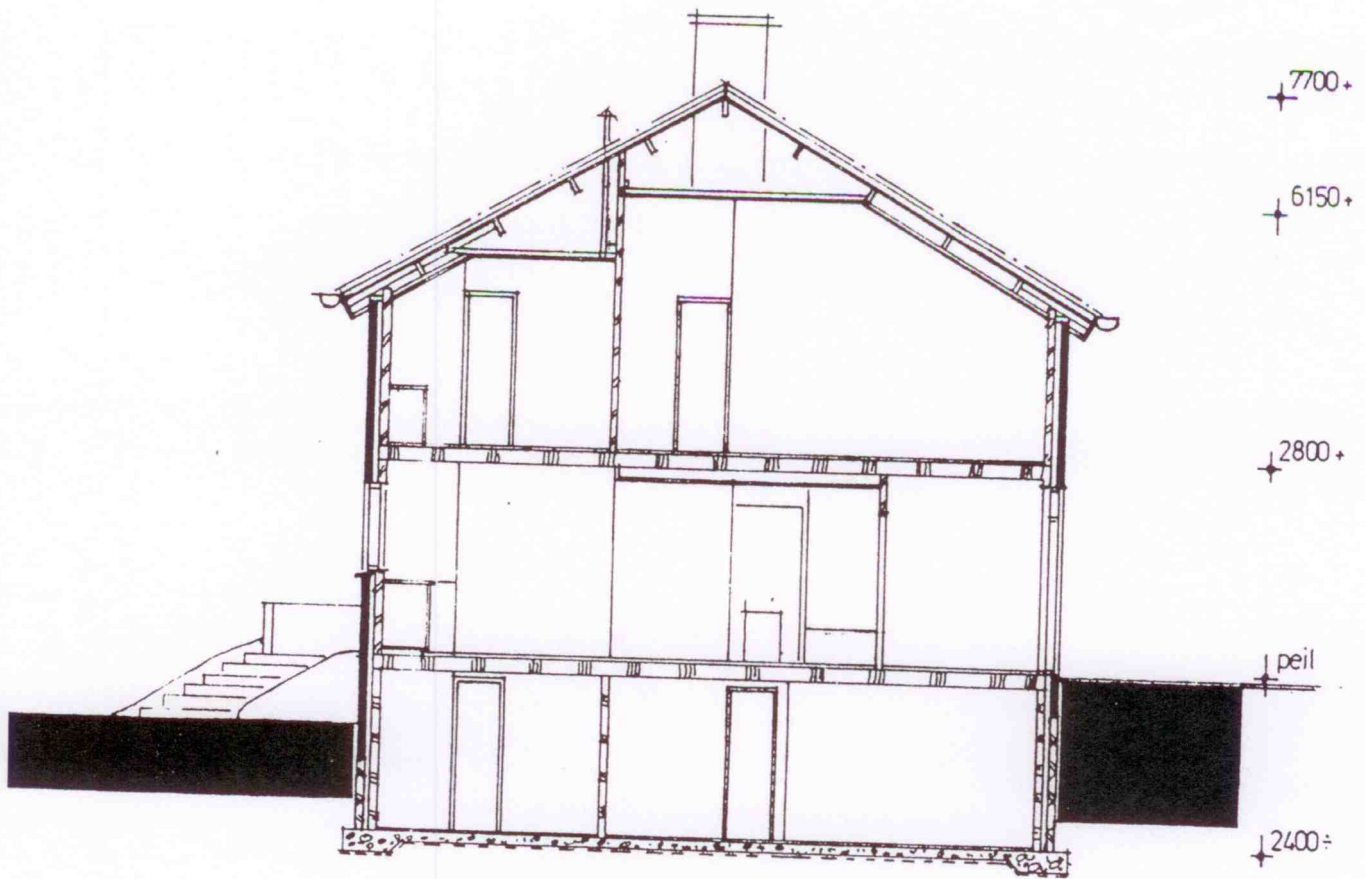
doorsnede b-b
